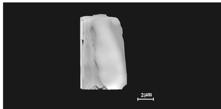
“嫦娥石”真实颗粒CT扫描三维形态图(2022年9月)。新华社发
