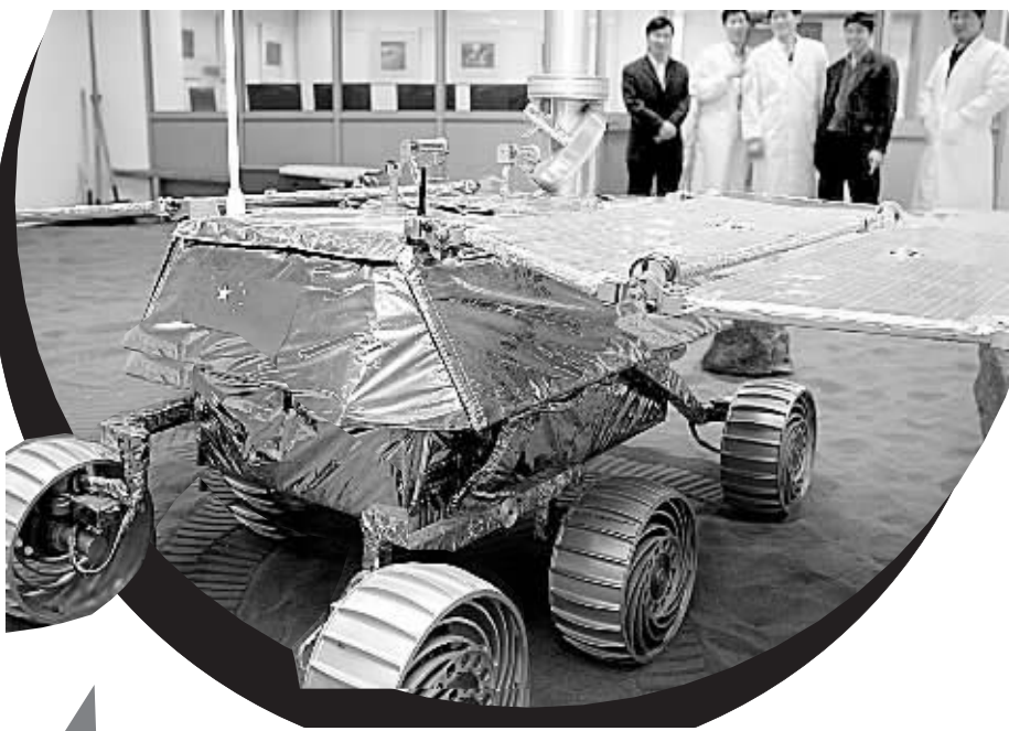
由上海航天局联合国内数十家科研机构共同研制的月面巡视探测器通常被称为“月球车”,它是我国“绕、落、回”三步走探月工程中,实现第二步“落”的重要部分。MR-2月球车采用独立驱动的六轮摇臂式行走系统,可爬越30度斜坡,跨越25厘米障碍。行进速度为每小时100米,最快可达每秒5厘米。新华社发
