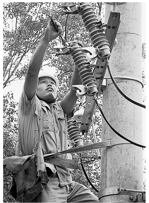
近日,唐庄供电所职工认真落实“井井通”工程,通过省电力公司划拨、登封市电业公司配套、当地群众自筹等方式筹资50万元,经过近两个月的艰苦作业,彻底解决了该乡范家门、塌上、雨台三个村浇地难问题。图为供电所职工在关帝庙村变电站施工。 李焱 王晓慧 摄
