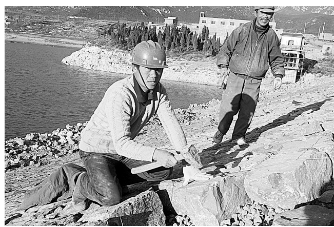
总投资1080万元的马庄水库除险加固工程,自今年8月份开工以来各项工作进展顺利,截至目前已经完成总工程量的80%,预计12月底将全部竣工。 通讯员 王晓慧 摄
