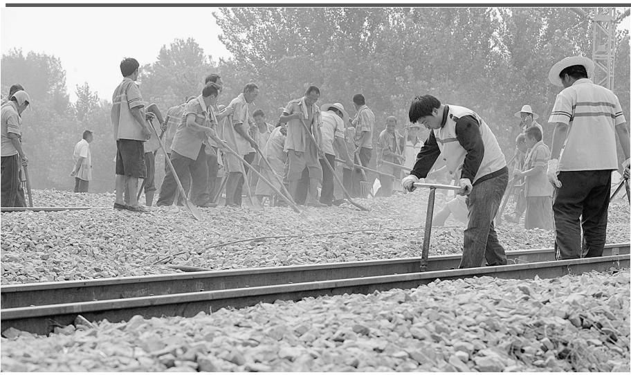
昨日,在位于惠济区古荥铁路寨的京广铁路线上,近百名铁路维修工正在回填石子固定铁轨。据介绍,该工程属于西绕城京广线立交改造项目,此处由以前宽7米的单孔铁路立交,改造成宽50米的4孔铁路立交。受施工影响,该路段火车通行只能减速慢行,时速在40公里左右。目前,该工程进入收尾阶段,工人们正在加紧施工,确保本月18日能够恢复正常通车。 本报记者 李利强 摄
