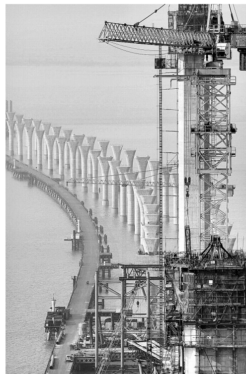
建设中的浙江嘉(兴)绍(兴)跨江大桥进展顺利,最高的主墩塔架施工高度已超过120米。嘉绍跨江大桥是杭州湾上第二座跨江大桥,于2008年年底动工,预计2012年年底建成通车。届时,浙江绍兴到上海的车程将缩短近一半。 新华社发
