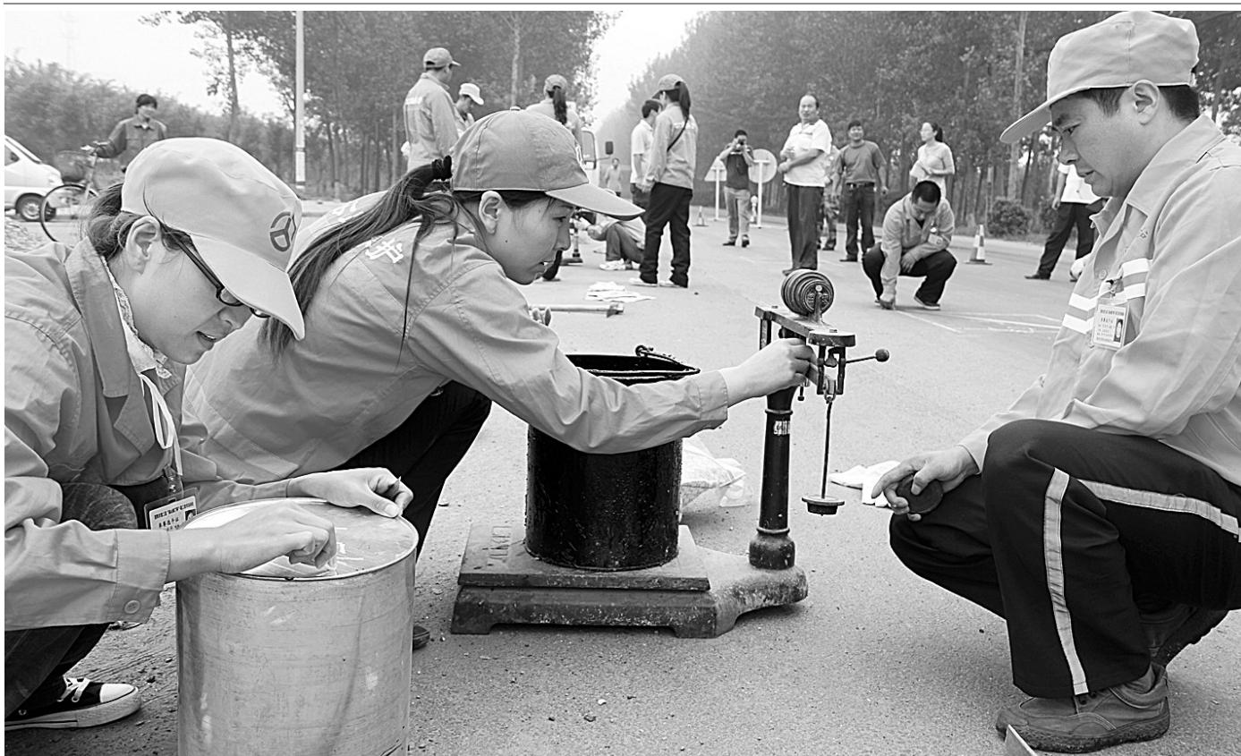
为提高道路养护水平,近日,荥阳市交通局举行了道路养护技术大比武。此次技术比武共分6个小组,每组4个人,比武地点选在一条需要修补的乡道上。比赛要求在30分钟内各组将各自的1平方米的坑槽修补结束。图为参赛人员正在称取桶的重量。
