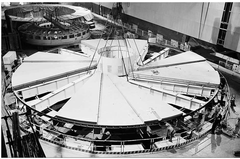
1月14日下午,世界上单机容量最大的首台80万千瓦水轮发电机组上机架在向家坝水电站右岸地下厂房顺利吊装就位,预计2012年并网发电。这是金沙江向家坝1号水轮发电机组上机架吊装现场。
