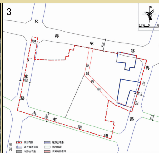
3. 道路系统规划图
