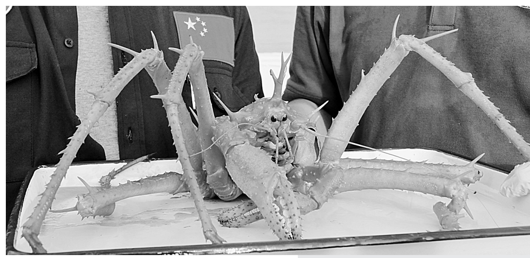
这是“蛟龙”号载人潜水器在南海一冷泉区采集到的蜘蛛蟹(6月19日摄)。
