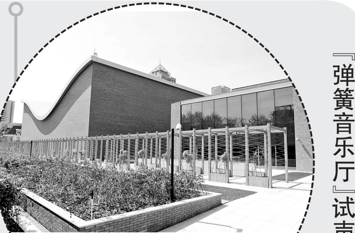
4月15日中国首座全部建造在弹簧隔振器上的音乐厅——上海交响乐团音乐厅首次对媒体和公众开放,并进行了声学试验。这座“弹簧音乐厅”外观仿佛是一个巨大的“马鞍”,内部包含一个可容纳1200名观众的演奏大厅和一个可容纳400人的室内乐演奏厅。
