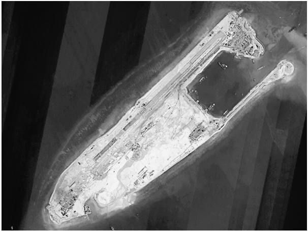
完成陆域吹填工程后的永暑礁卫星图片。新华社发
