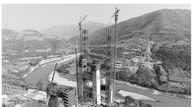
24日,中缅国际铁路大理至瑞丽段的控制性工程——怒江特大桥全面开工。位于云南省施甸县与龙陵县交界处的怒江特大桥主跨采用跨度达490米的钢桁拱梁,是目前世界上跨度最大的钢桁梁铁路拱桥。 新华社发
