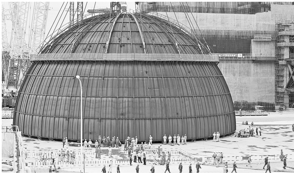
“华龙一号”采用了多项先进安全理念,抗9级地震,防大型海啸,并且设计了一套非能动安全系统,在发生极端灾难时,即便失去外部电源,依然能够保证核反应堆安全。
