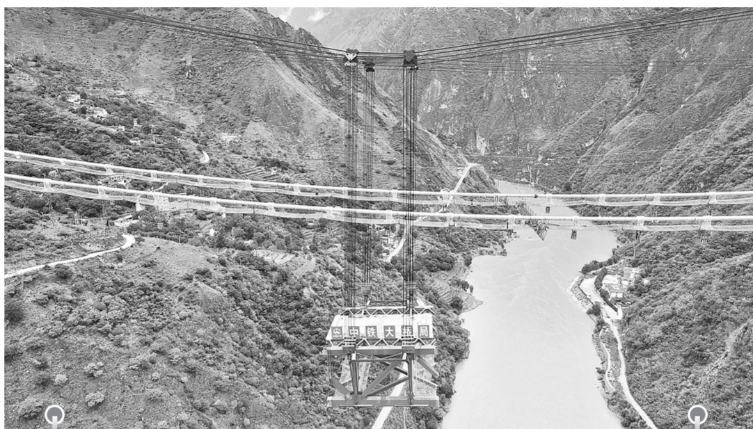
6月15日，缆索吊机在吊装钢桁梁。当日，随着缆索吊机将长24.4米、高12米、重640吨的钢桁梁平稳固定在吊索上，由中铁大桥局承建的丽(江)香(格里拉)铁路金沙江特大桥首片中跨钢桁梁架梁成功。新华社发
