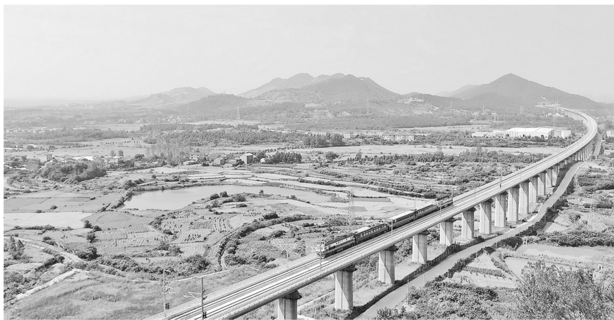
9月16日,首趟检测列车行驶在安九高铁线路上。当日,安九高铁安庆至黄梅段开始联调联试,为全线开通运营奠定基础。安九高铁连接安徽省安庆市与江西省九江市,是国家中长期铁路网规划“八纵八横”高速铁路主要通道京港(台)通道的重要组成部分,设计时速350公里。 新华社发
