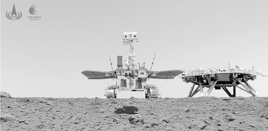
这是“着巡合影”图。2021年6月11日，国家航天局在北京举行天问一号探测器着陆火星首批科学影像图揭幕仪式，公布了由祝融号火星车拍摄的着陆点全景、火星地形地貌、“中国印迹”和“着巡合影”等影像图。
