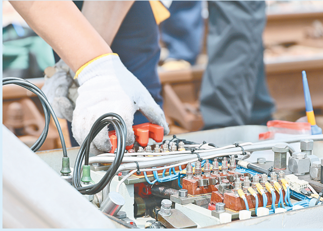
郑州高铁基础设施段内，工作人员顶着烈日进行道岔检修作业
